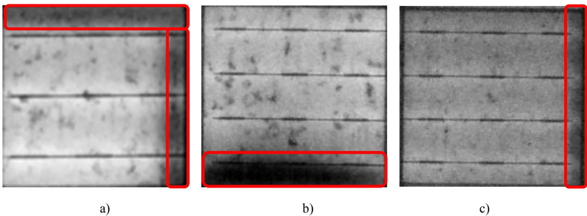
a) b) c) 图 D. 16 黑边的图像
