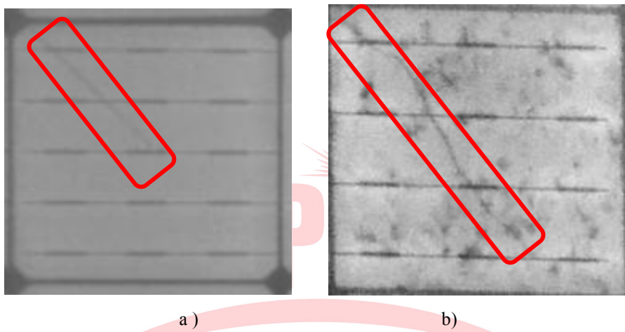
图 D.4 与焊带成 45^\circ 的微裂纹图像
