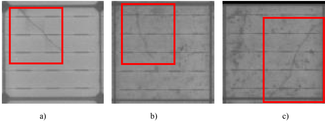
图 D.3 非贯穿的微裂纹图像
