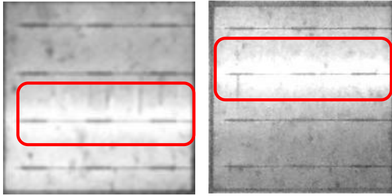
a) b) 图 D. 14 亮斑的图像
