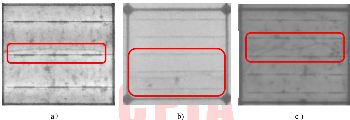
图 D.1 平行于焊带的微裂纹图像
