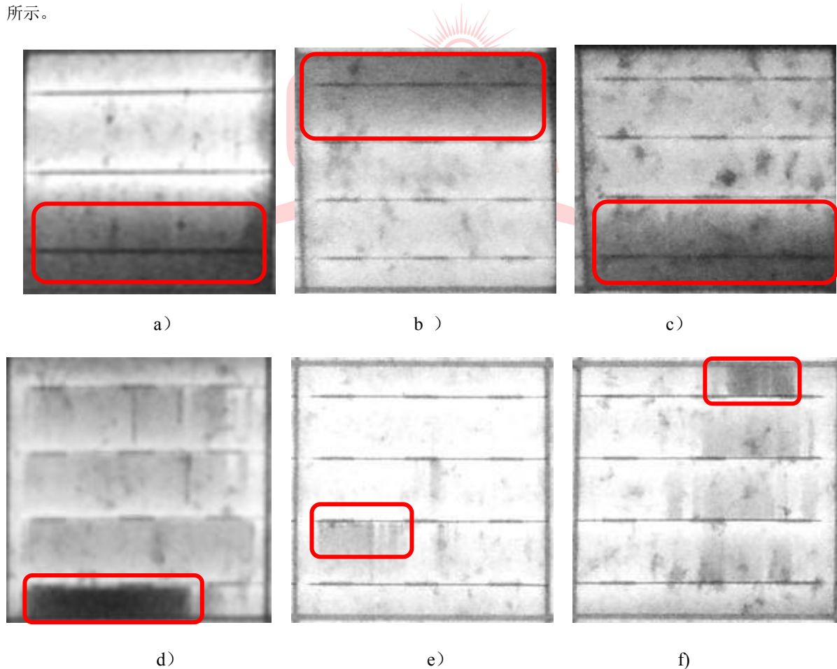
图 D. 13 暗斑的图像
