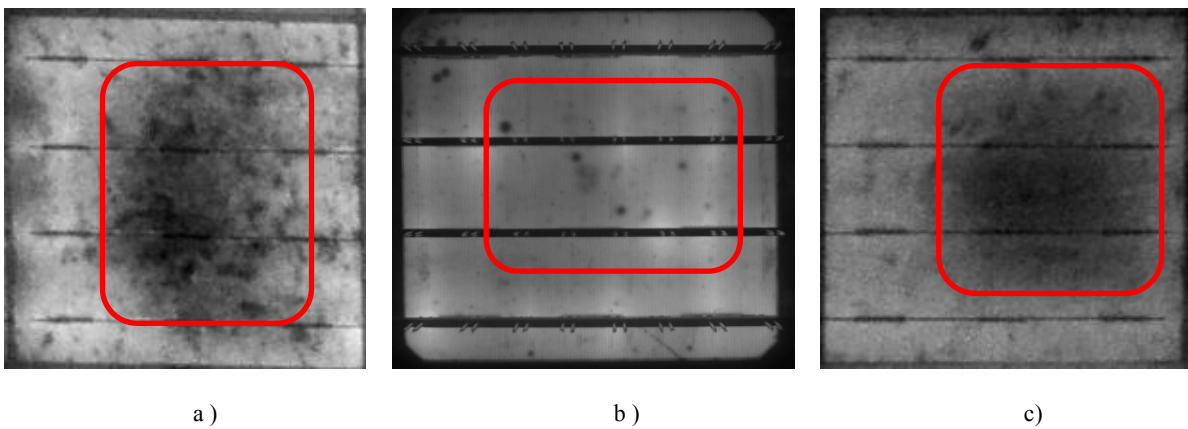
图 D. 8 黑斑的图像
