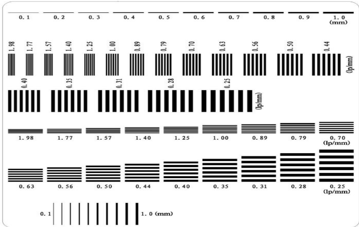
C.1 校准样板示例
