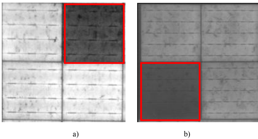
图 D.11 失配的图像
