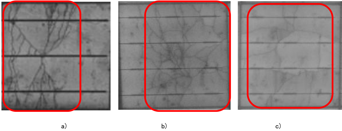
图 D. 6 脉状的微裂纹图像
