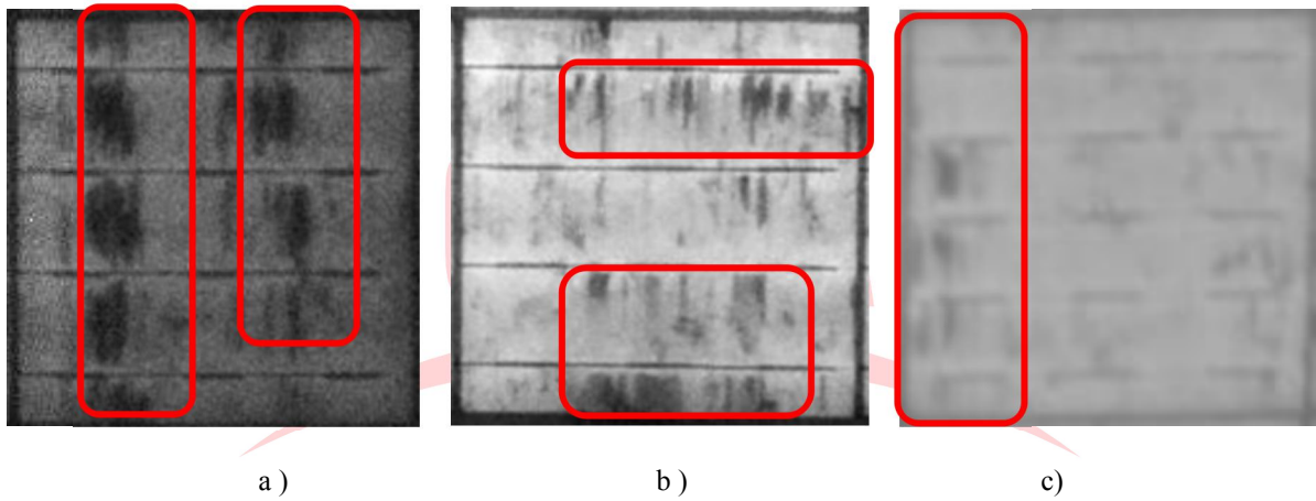
a) b) c) 图 D. 15 断栅的图像
