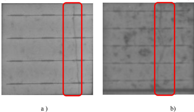
图 D.2 垂直于焊带的微裂纹图像
