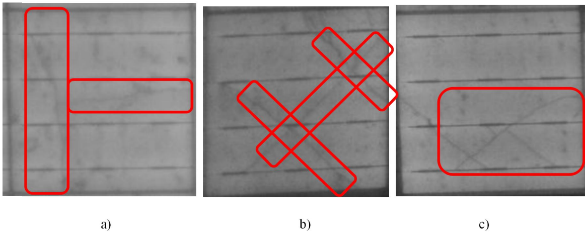
图 D.5 交叉的微裂纹图像
